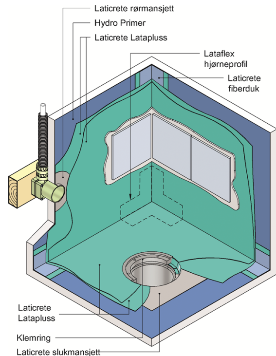
Fig. 1 viser oppbygning av Latapluss membransystem
